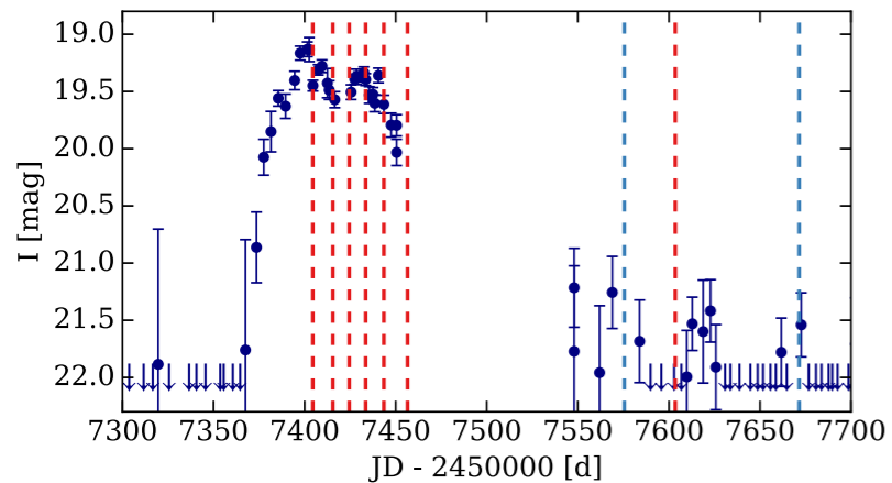
OGLE16aaa TDE
